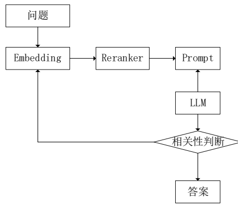
图 4 自适应检索
