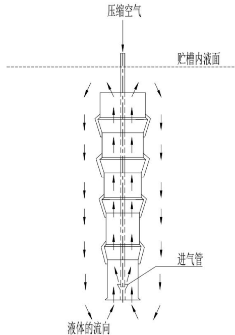
图 2 空气升液循环器示意图
