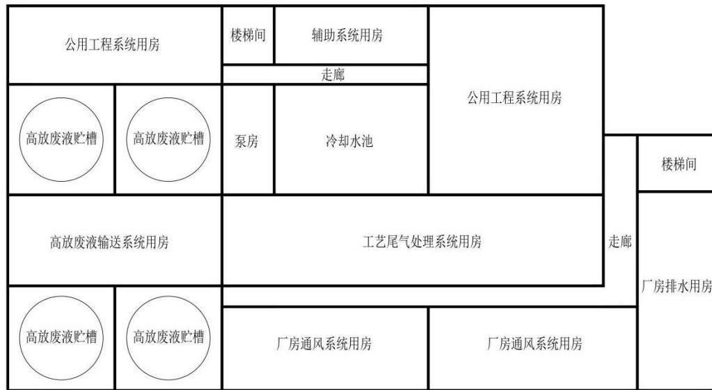
图 4 高放废液贮存厂房地下部分平面图
