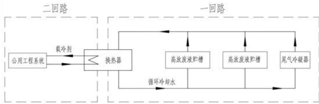
图 1 高放废液循环冷却水系统示意图
